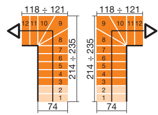
Deckenloch
